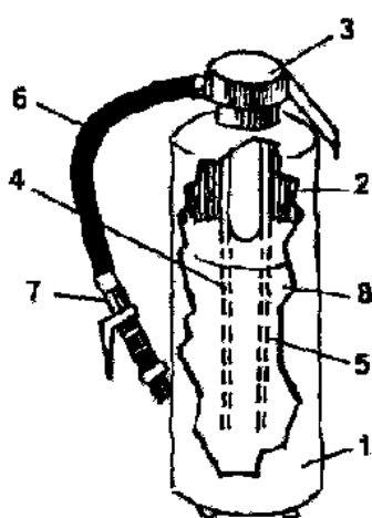
Рис.8.5. Порошковый огнетушитель:
