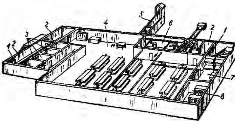
Рис.16.1. План убежища:
